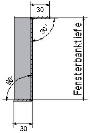
B-B ( 3 : 4 )
